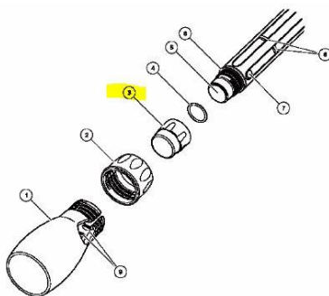
Rysunek 2. Widok końcówki elektrody
